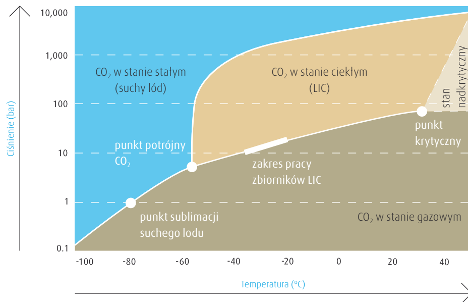
Wykres fazowy dla dwutlenku węgla
